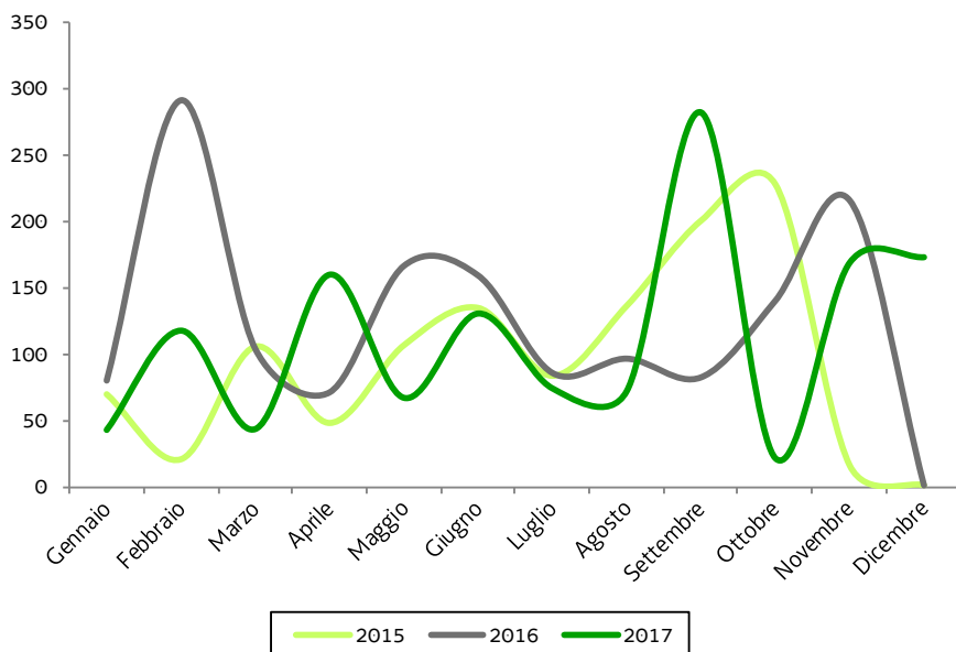
Graf. 2.2 - FVG PRECIPITAZIONI CUMULATE (millimetri) - Anni 2015-2017
