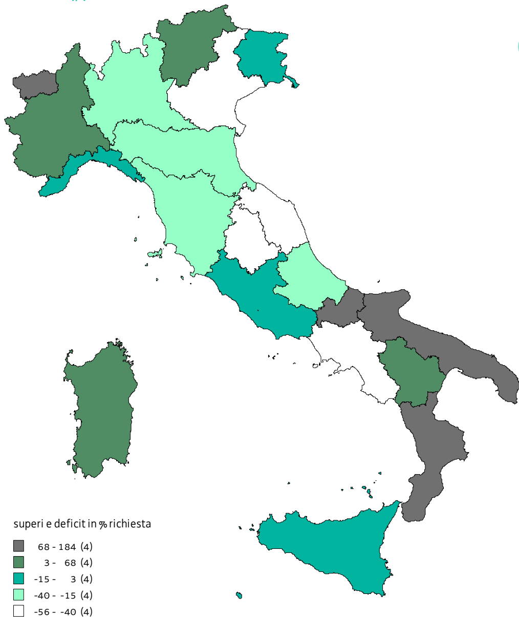
Cart. 5.1 - ITALIA SUPERI E DEFICIT DELLA PRODUZIONE DI ENERGIA ELETTRICA RISPETTO ALLA RICHIESTA (%) - Anno 2017
