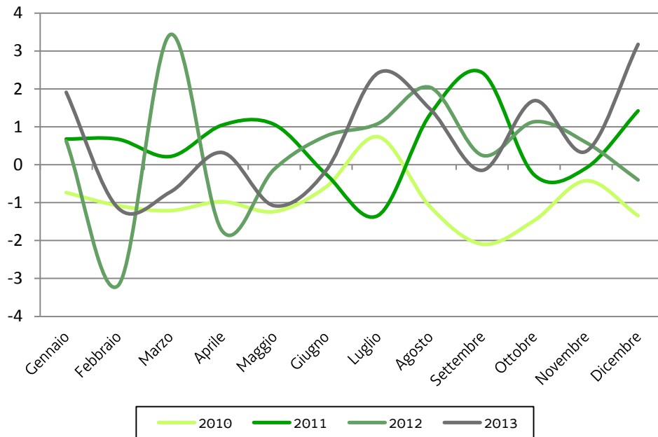
Graf. 2.1 - FVG TEMPERATURA MEDIA MENSILE: ANOMALIE (differenza in °C. rispetto alla media mensile dei 10 anni precedenti)
