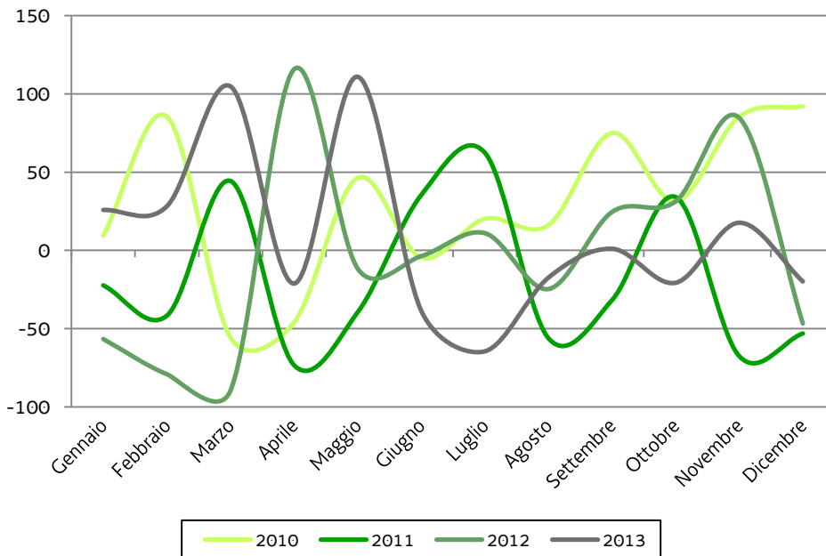
Graf. 2.2 - FVG PRECIPITAZIONI CUMULATE: ANOMALIE (differenza % mensile rispetto alla media mensile dei 10 anni precedenti)
